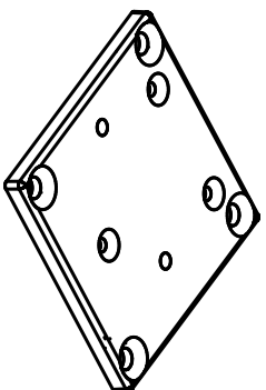
(A): Durchgangsloch mit Kegelsenkung für M2.5-Schraube
