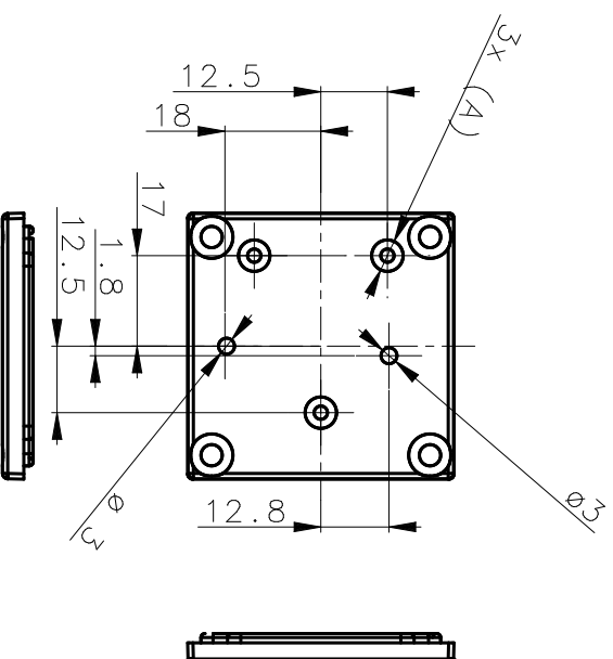
(A): Durchgangsloch mit Kegelsenkung für M2.5-Schraube
