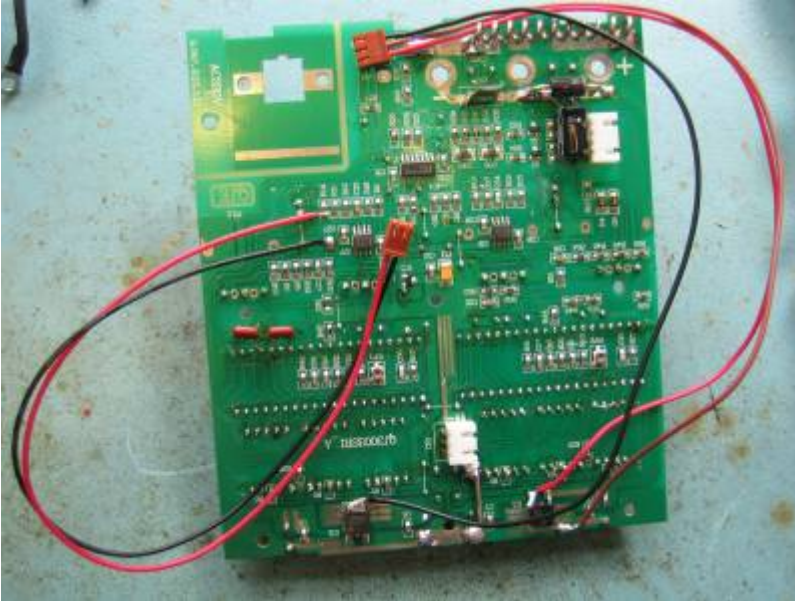
JAE-Kabel anlöten
