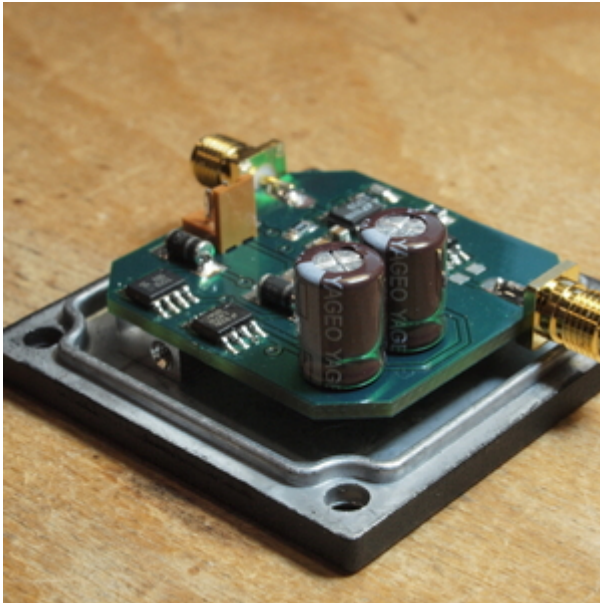
sagatrigger_04.jpg
