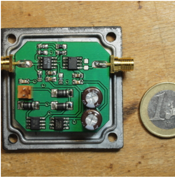
sagatrigger_01.jpg
