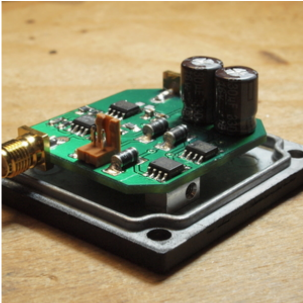
sagatrigger_02.jpg
