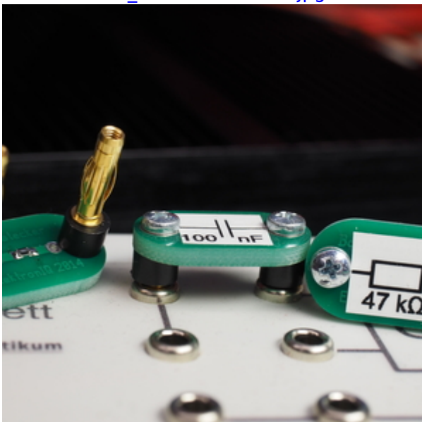
bauteilstecker_buchsenbruecke.jpg
