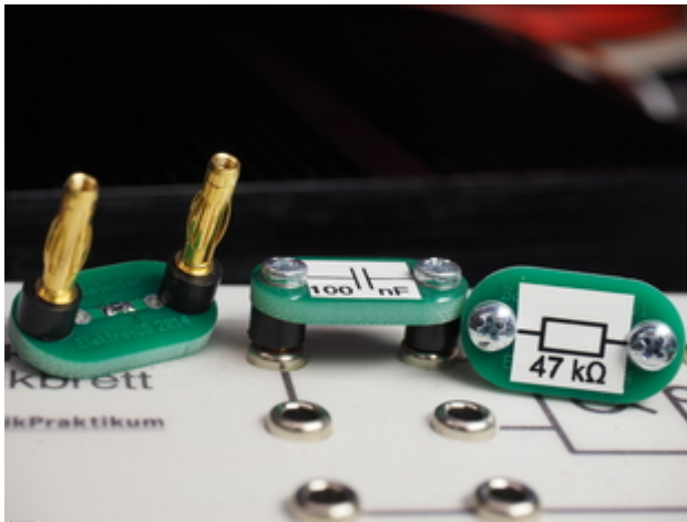
BauteilStecker
