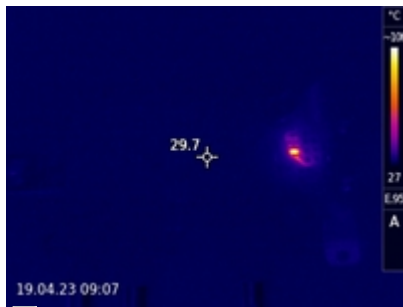
Ein falscher Transistor im Wärmebild
