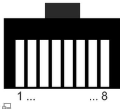
RJ45, Sicht auf den Stecker
