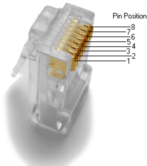
RJ45-Stecker. (Lizenz: GPL 1.2 )
