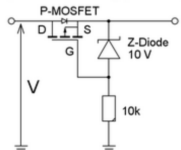
positive Spannung ( V > \text{GND} )
